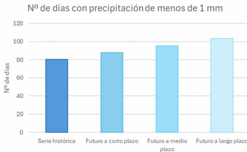
Figura 39. Diagrama de variación del número de días al año en los que se registran en El Palmar de Troya valores de precipitación inferiores a 1 mm para la serie histórica de 1961 a 1990 y para los horizontes temporales de futuro a corto, medio y largo plazo.
