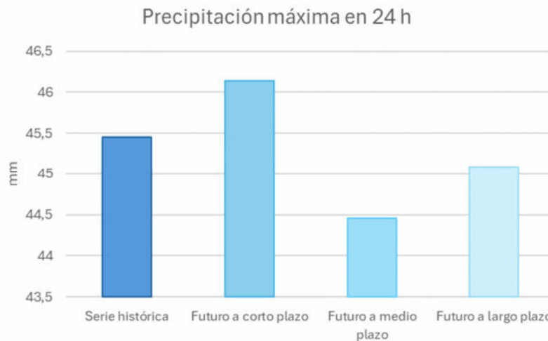
Figura 40. Diagrama de variación de los valores de precipitación máxima en 24 h en El Palmar de Troya para la serie histórica de 1961 a 1990 y para los horizontes temporales de futuro a corto, medio y largo plazo.
