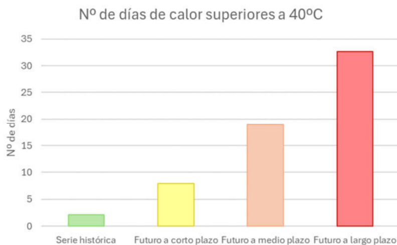
Figura 36. Diagrama de variación del número de días en los que se superan los 40°C al año en El Palmar de Troya para la serie histórica de 1961 a 1990 y para los horizontes temporales de futuro a corto, medio y largo plazo.
