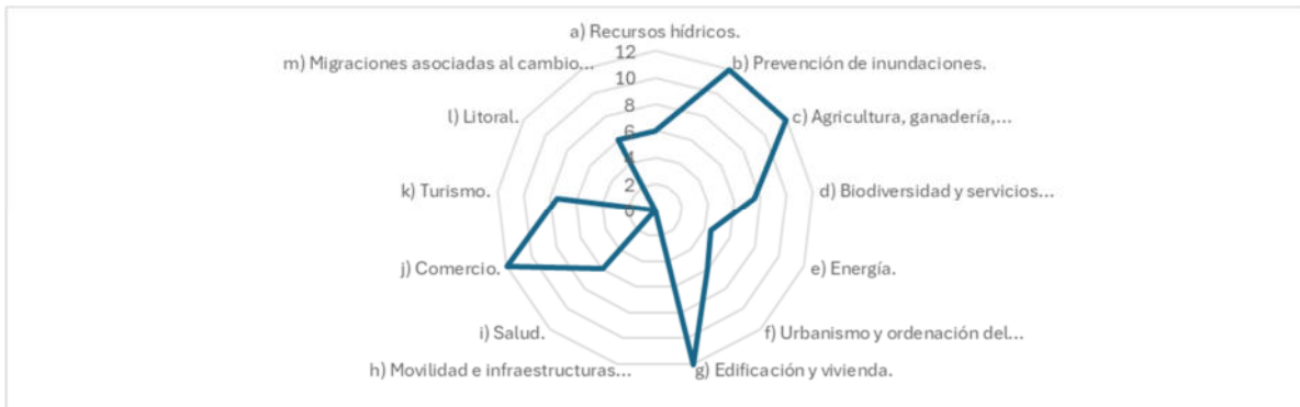
Figura 46. Diagrama resumen de las valoraciones del riesgo del impacto "cambios de la disponibilidad del recurso agua y pérdida de calidad" en las áreas estratégicas seleccionadas en El Palmar de Troya.
