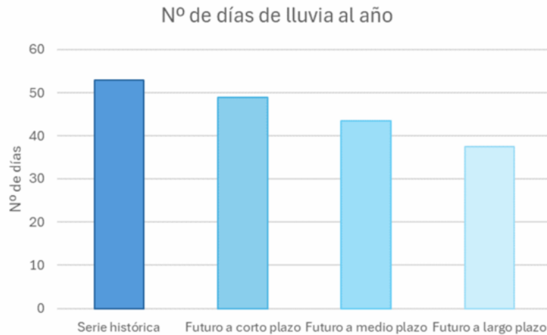
Figura 38. Diagrama de variación del número de días al año en los que llueve en El Palmar de Troya para la serie histórica de 1961 a 1990 y para los horizontes temporales de futuro a corto, medio y largo plazo.
