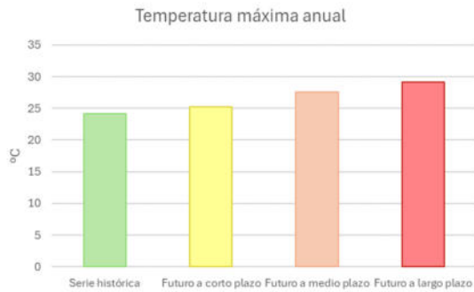
Figura 35. Diagramas de variación de las temperaturas media (izquierda) y máximas (derecha) anuales en El Palmar de Troya para la serie histórica de 1961 a 1990 y para los horizontes temporales de futuro a corto, medio y largo plazo.
