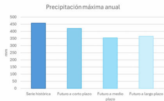
Figura 37. Diagramas de variación de los valores de precipitación media (izquierda) y máxima (derecha) anuales en El Palmar de Troya para la serie histórica de 1961 a 1990 y para los horizontes temporales de futuro a corto, medio y largo plazo.
