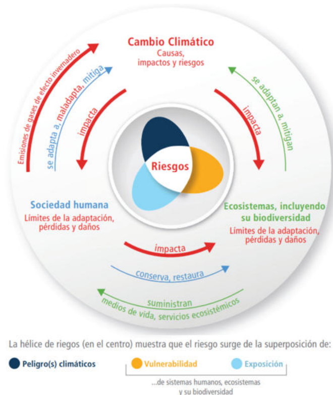
Figura 34. Cambio Climático: esquema de causas, impactos y riesgos.
